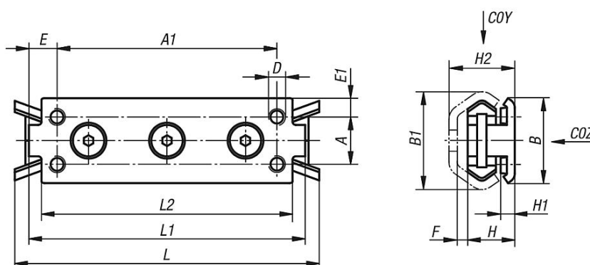
Festlager Kompaktausführung
