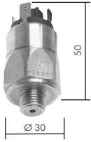
Druckschalter
